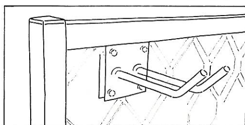
Exempel på montering av redskapskonsoll
